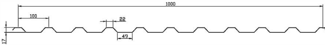
Profilgeometri KAMI TP
